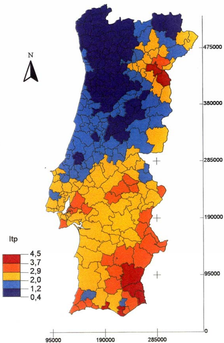
Figura 18 - Amplitude térmica.
